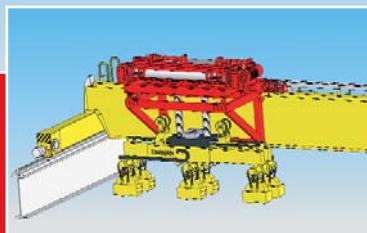
Jeřáb GKMJ 14,5t/22,4m s lanovou stabilizací a magnety na roznášecí traverze.
