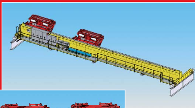
Jeřáb GKMJ 10+10t/25,4m s lanovou stabilizací a magnety na roznášecích traverzách.
