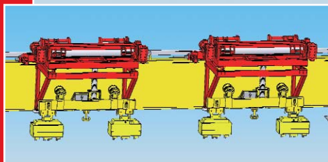
Jeřáb GKMJ 10+10t/25,4m s lanovou stabilizací a magnety na roznášecích traverzách.
