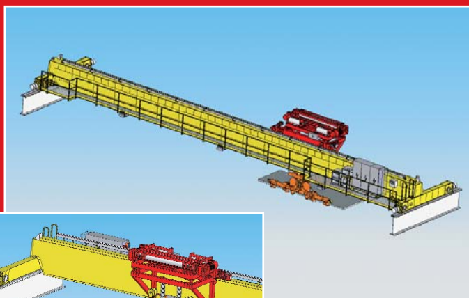
Jeřáb GKMJ 14,5t/25,4m s lanovou stabilizací a kleštěmi na plechy.
