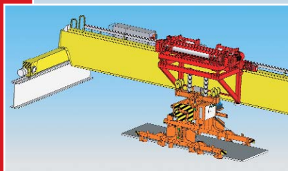
Jeřáb GKMJ 14,5t/25,4m s lanovou stabilizací a kleštěmi na plechy.
